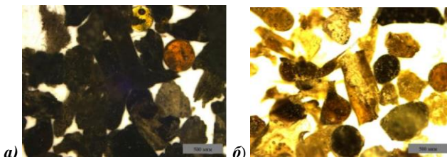
Рис. 1 Форма частиц отходов производства минеральной ваты ООО «Комбинат теплоизоляционных изделий» (г. Саранск) фракций: a – 0,63...1,25; б – 0,315...0,63
