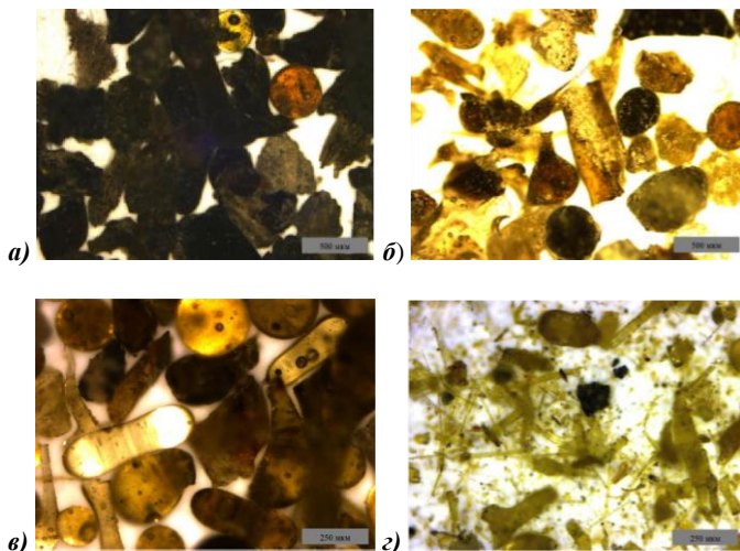
Рис. Форма частиц отходов производства минеральной ваты ООО «Комбинат теплоизоляционных изделий» (г. Саранск) фракций: а – 0,63...1,25; б – 0,315...0,63; в – 0,16...0,315; г – поддон
